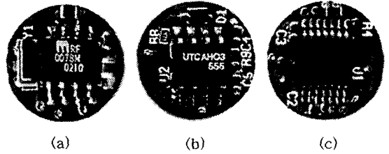
그림 3. 구현된 초소형 PCB 모듈; (a) 수신 및 디코더부, (b) 펄스 발생부, 및 (c) 출력부
