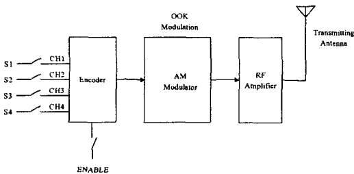
그림 2. 캡슐 제어용 송신기의 블록 다이어그램
