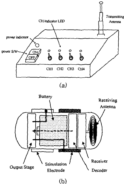
그림 1. (a) 캡슐 제어용 송신기 및 (b) 자극용 캡슐
