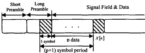
<그림 7> SFBC 기법을 위한 frame 구조
