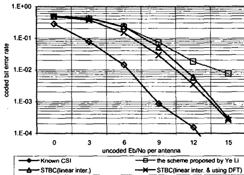
<그림 10> 150ns RMS delay 를 가지는 exponential decaying fading 에서 STBC 기법을 통해 추정된 채널 계수에 의한 성능 곡선
