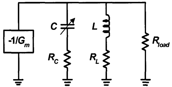
그림 5. LC-VCO의 동가회로
