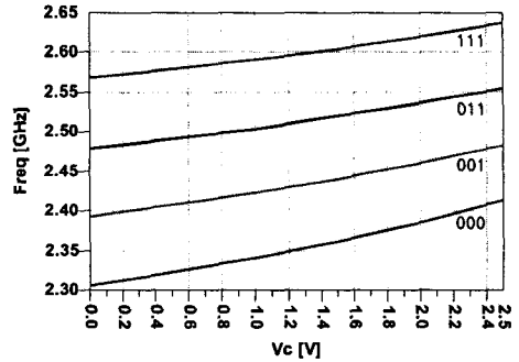
그림 8. 입력전압 V_c 에 따른 발진주파수 범위
