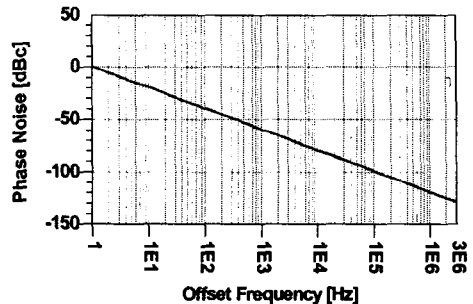
그림 9. 위상잡음
