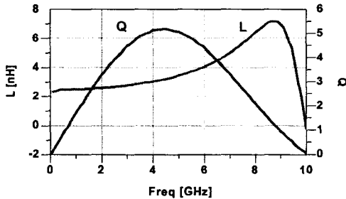
그림 7. 설계된 인덕터의 Q와 인덕턴스 L
