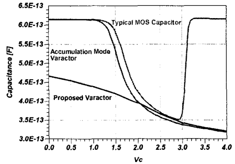
그림 3. 일반적인 MOS 바랙터, 축적모드 바랙터, 제안된 바랙터의 동작영역
