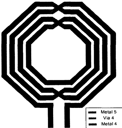
그림 4. 8각 나선형 인덕터
