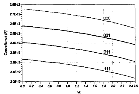
그림 3. 3-bit 디지털 튜닝과 아날로그 튜닝 조합으로 구현된 커패시턴스 특성 곡선
