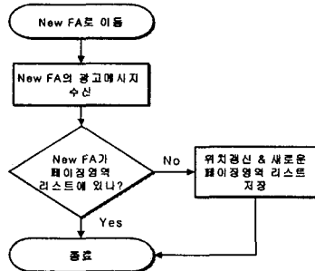
그림 2. 단말에서의 위치등록 알고리즘 순서도
