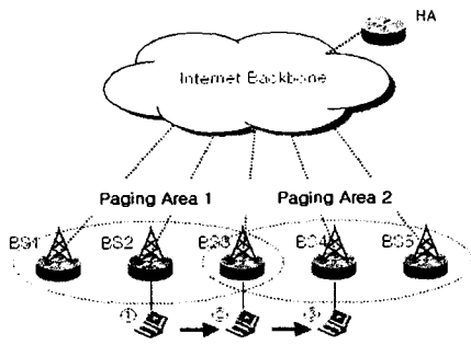
그림 1. 제안하는 페이징영역 구조
