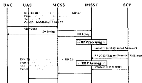
그림 3. 080 지능망 서비스 예
