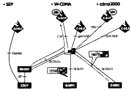
그림 2. 통합된 서비스 처리 구조
