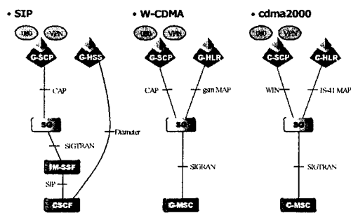
그림 1. 각 방식 별 서비스 처리 구조
