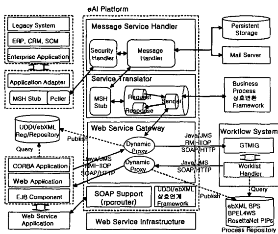
그림 4 eAI 플랫폼 구성도
