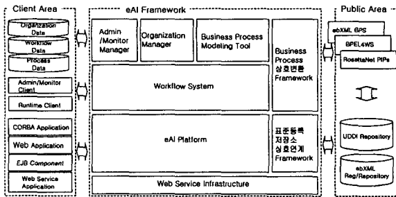
그림 1 eAI 프레임워크 구성도
