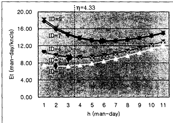
그림 2) 코드검증 공수(h)에 따른 결함 수정 총공수(Et)
