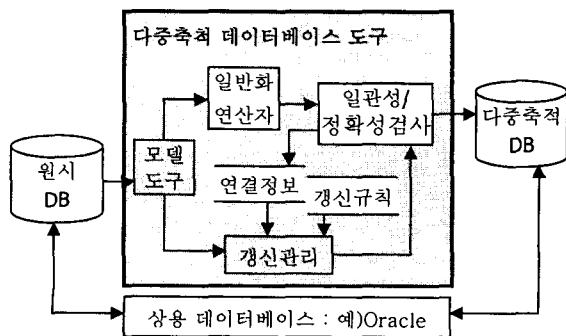
그림 1. 다중축척 데이터베이스를 위한 시스템 구조
