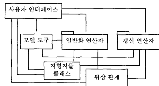
그림 2. 패키지 다이어그램
