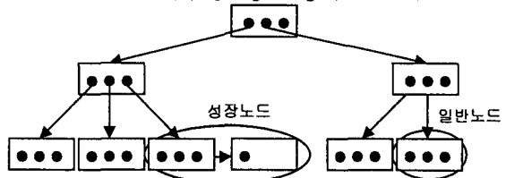
그림 1 성장 노드
