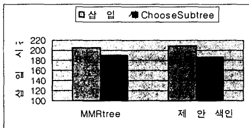
그림 2 삽입 시간
