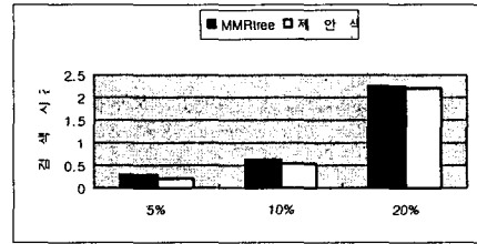
그림 3 검색 시간
