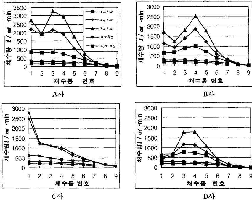
Fig. 8. 원형 헤드의 살수분포
