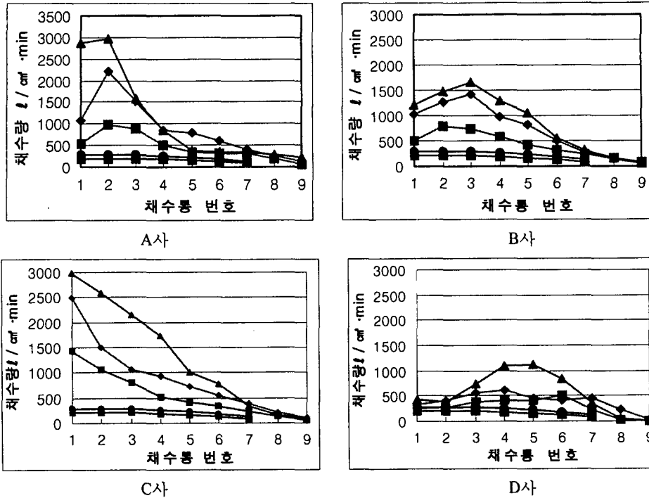
Fig. 9. 하향형 헤드의 살수분포
