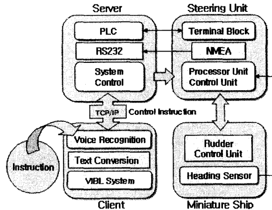
그림 6. 원격 조타기 제어 시스템 구성
