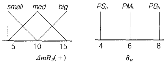
그림 5. \Delta mR_\theta(+) 과 \delta_u 의 멤버십함수
