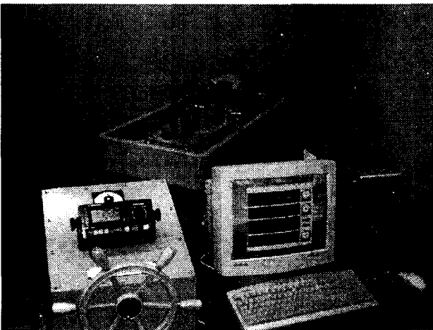
그림 7. 모형 선박 시스템 구성
