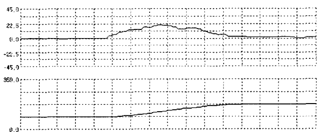
(a) 자동조타기(FURUNO FAP-330)
