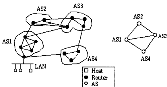
(a) 라우터 계층 (b) AS 계층 (그림 1) 인터넷 위상
