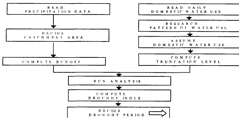
그림 2. DDP 모형을 단순화한 순서도
