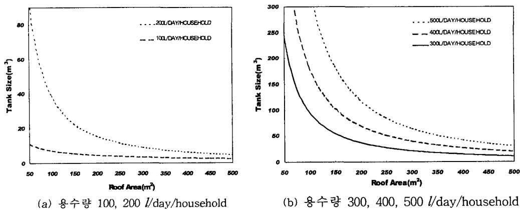
그림 4. 우수이용 시스템의 설계
