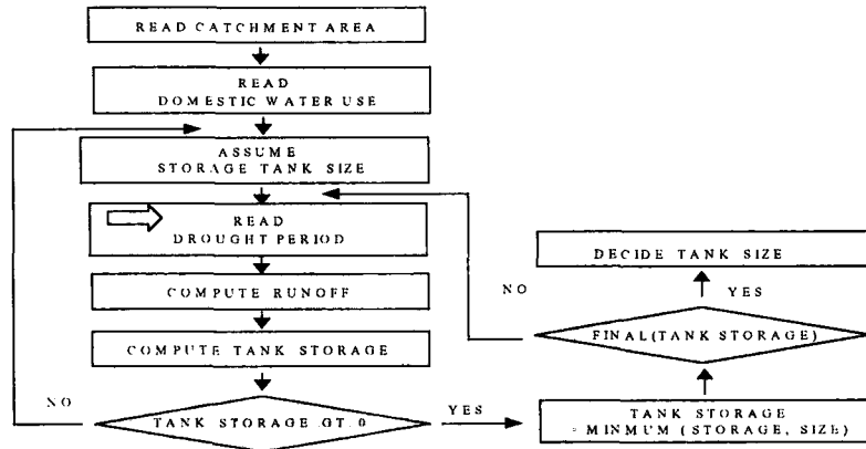
그림 3. DOS 모형을 단순화한 순서도
