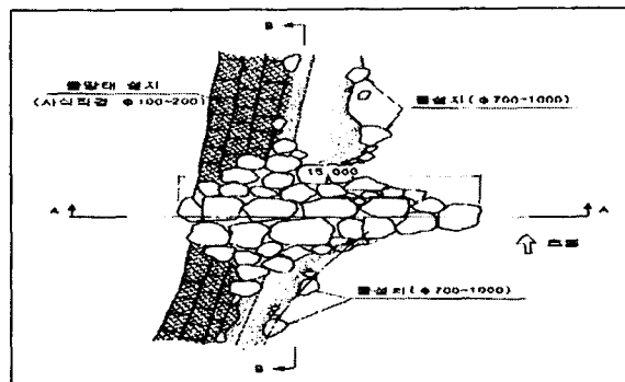
평면도
