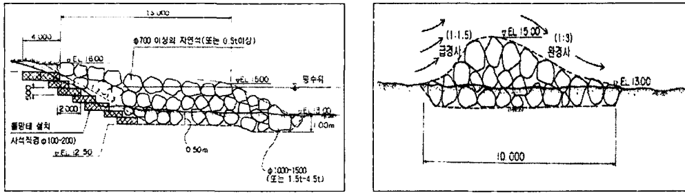
A-A 단면
