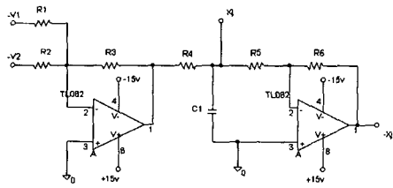
그림 4. CNN 회로도 Fig. 4 CNN circuit
