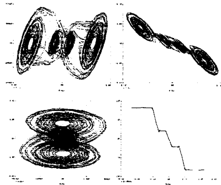
그림 5. 송신부 SC-CNN의 2-double scroll 어트랙터 그리고 비선형출력 Fig. 5 Attractor of 2-double scroll of SC-CNN and nonlinear output according to x_1
