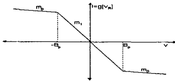
그림 2. 비선형 저항의 전압 전류 특성 Fig. 2 v-i characteristic of nonlinear resistor
