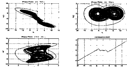
그림 3. 2-double scroll 위상공간과 비선형 저항 Fig. 3 phase plane of 2-double scroll and nonlinear resistor
