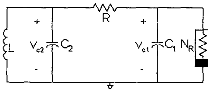
그림 1. Chua 회로
