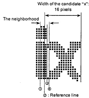
Figure 3. 집합 문자의 분할 비용(라인 ①의 분할 비용은 22, 라인 ②의 분할 비용은 21, 라인 ③의 분할 비용은 3, 라인 ④의 분할 비용은 3)
