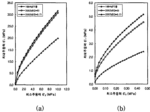
그림 7. Hoek-Brown 파괴기준 주응력 ( \sigma_1 - \sigma_3 ) 곡선
