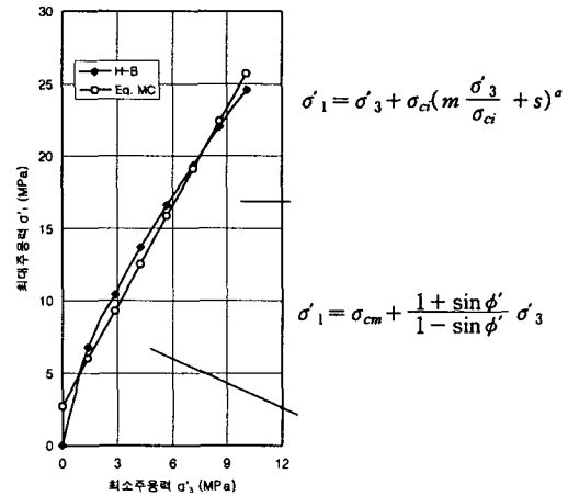
그림 1. 등가 Mohr-Coulomb Envelope
