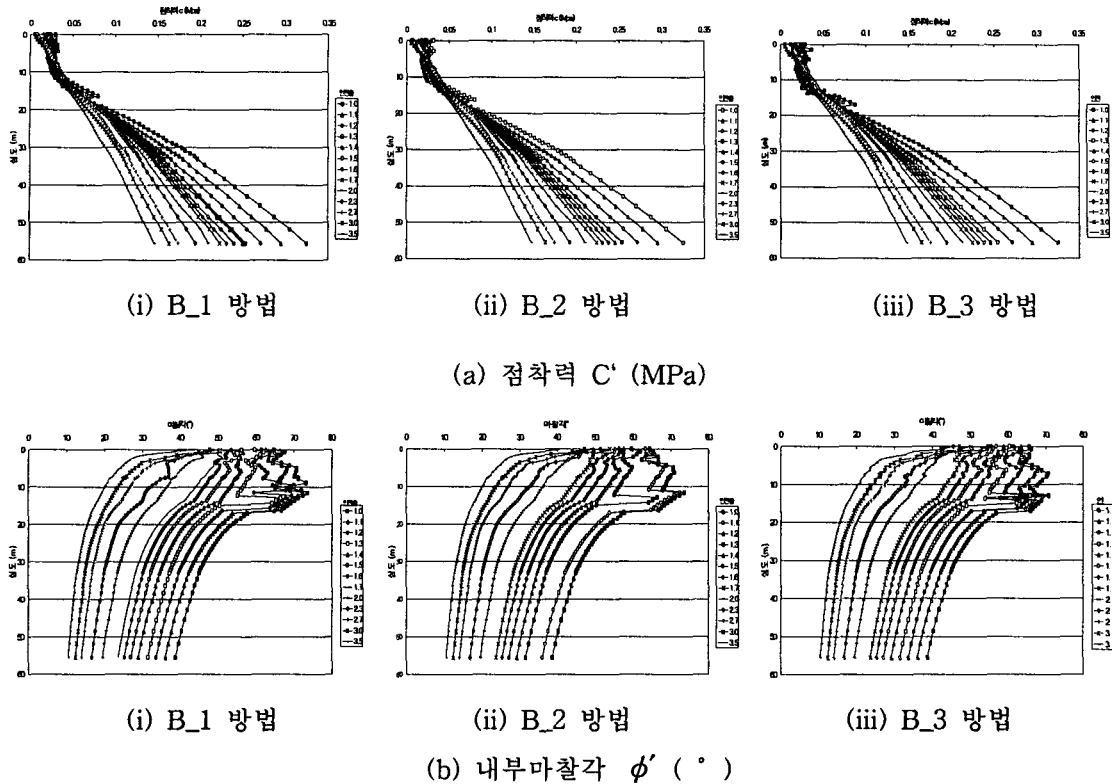
그림 6. 강도감소를 변화에 따른 심도별 암반 전단강도정수 변화 (B방법)
