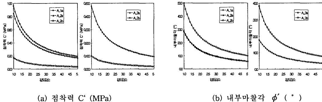
그림 5. 강도감소율 변화에 따른 암반 전단강도정수 변화 (A방법)
