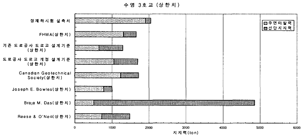
그림 3. 지지력 이론식값과 재하시험 실측값과의 비교(수영 3호교, 상한치)
