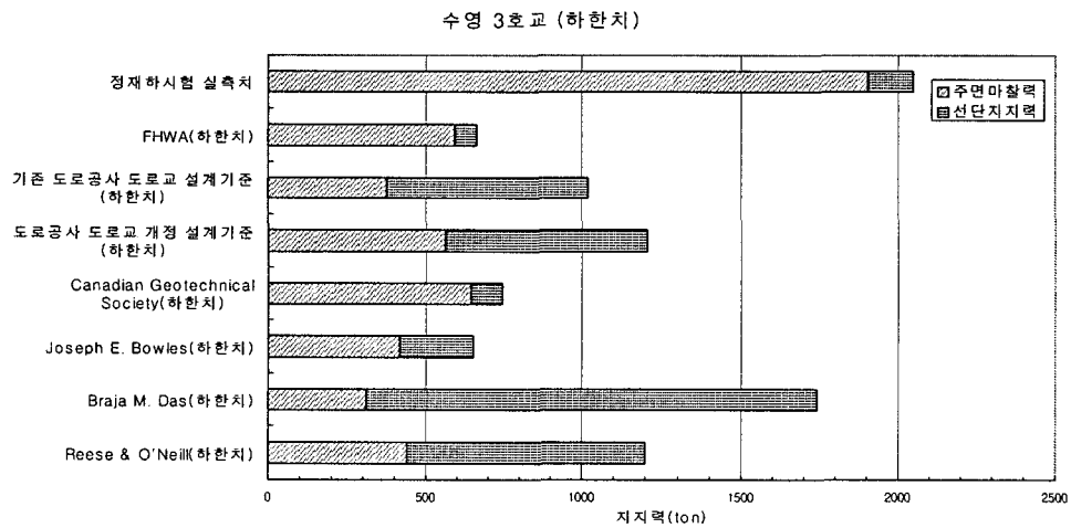
그림 4. 지지력 이론식값과 재하시험 실측값과의 비교(수영 3호교, 하한치)
