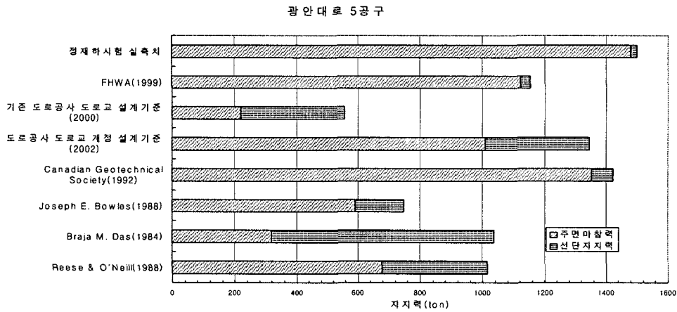
그림 2. 지지력 이론식값과 재하시험 실측값과의 비교(광안대로 5공구)
