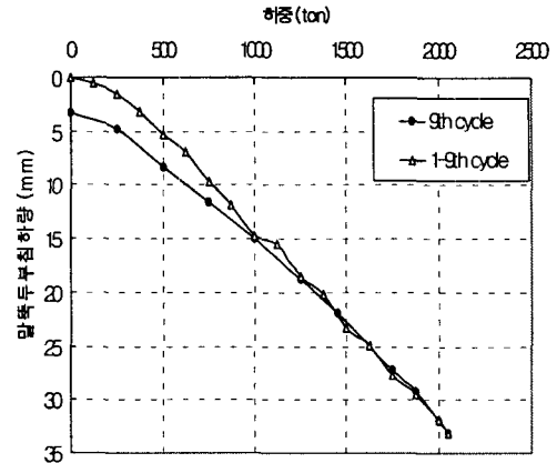
(b) 수영 3호교
