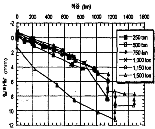
(a) 광안대로 5공구
