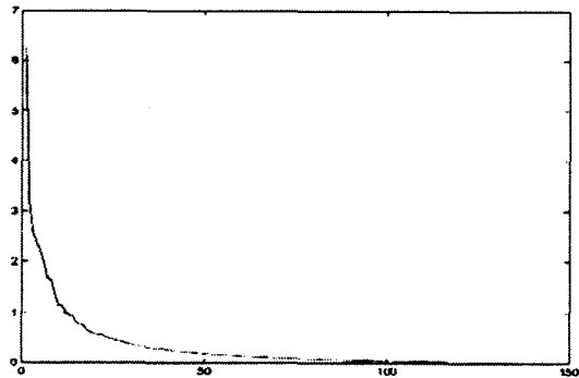
그림 6. PCA의 eigenvalues.
