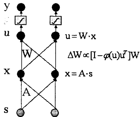
그림 1. ICA network 및 학습방법
