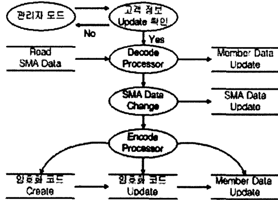
<그림 8> Data Update Processor
