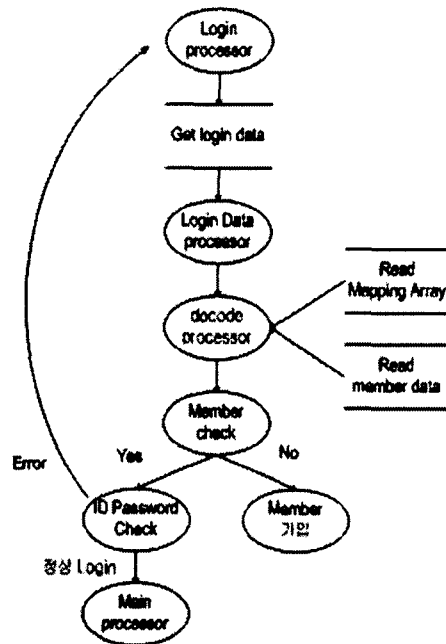
<그림 5> Login Processor
