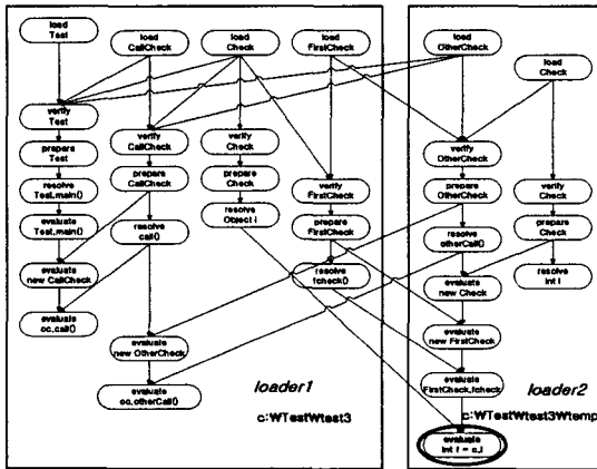
[그림 3-2] 클래스의 동작 분석
