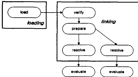
[그림 2-23] 자바 가상 머신의 동작
