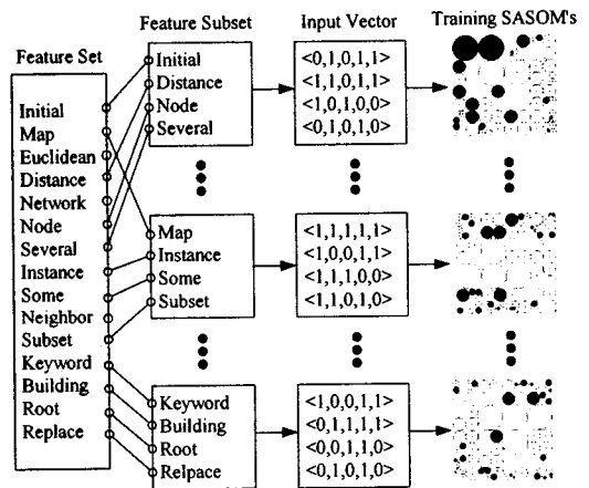
그림 3. 서로 다른 특징 집합을 사용한 SASOM 학습의 예
