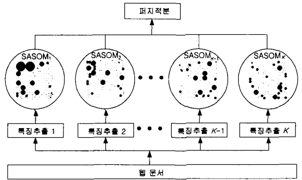
그림 1. 웹 문서 분류를 위한 다중 SASOM 분류기의 퍼지결합
