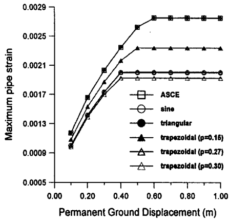
그림 5. 수정된 상호작용력을 이용한 비교해석
