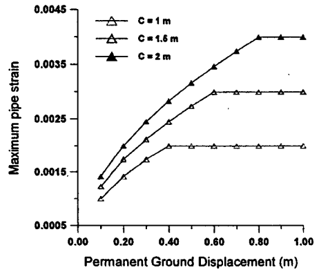
그림 8. 매설심도에 따른 해석(L=400m)
