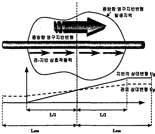
그림 2. O'Rourke 해석식의 개념도
