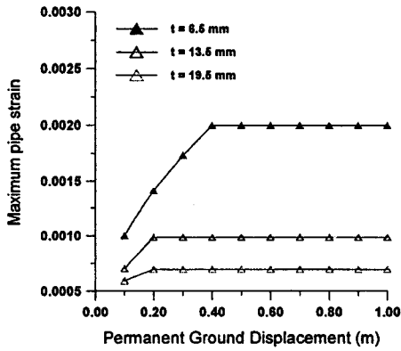
그림 7. 두께변화에 따른 해석(L=400m)
