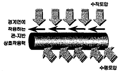
그림 3. ASCE 관·지반 상호작용력
