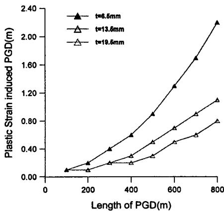
그림 9. 두께에 따른 한계지반변형의 변화
