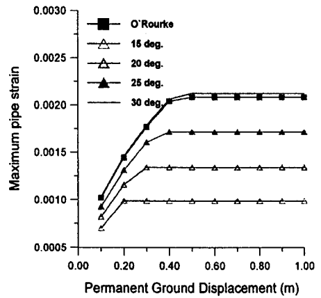
그림 6. 전단저항각 변화에 따른 해석
