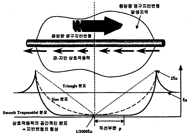
그림 4. 지반강성 감소를 반영한 관·지반 상호작용력의 산정
