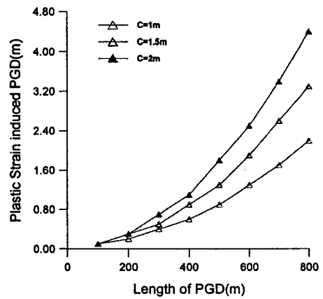
그림 10. 매설심도에 따른 한계지반변형의 변화
