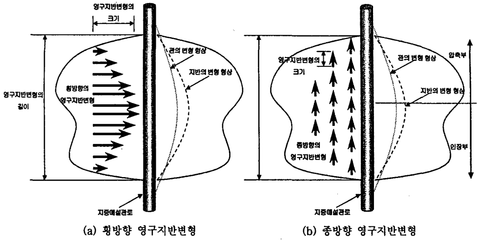
그림 1. 영구지반변형의 방향에 따른 매설관로 거동특성
