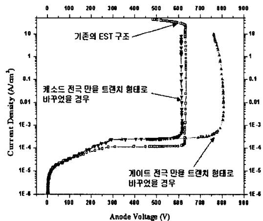
그림 3 기존의 EST와 제안한 EST소자의 순방향 저지 모드 시의 저지 전압
