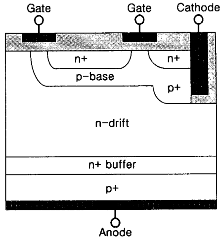
그림 1 (a) 기존의 EST (b) 제안한 EST(Type-1) (c) 제안한 EST(Type-2)
