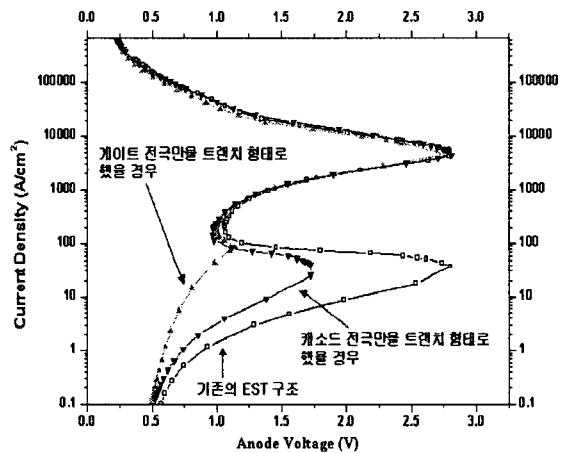
그림 2 기존의 EST와 제안한 EST의 순방향 전도 특성
