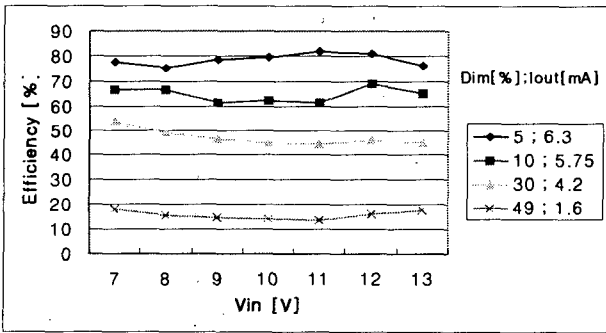
그림 9 인버터 효율(하프-브리지) Fig. 9 Inverter Efficiency by Vin and PW
