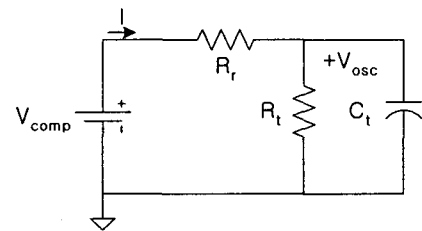
그림 6 VCO 설정 Fig. 6 Programming of the VCO
