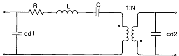
그림 3 압전 변압기의 등가회로 Fig. 3 Equivalent Circuit of PT
