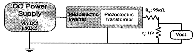
그림 7 압전 인버터 효율 측정 시스템 Fig. 7 Measurement System for Piezo Inverter
