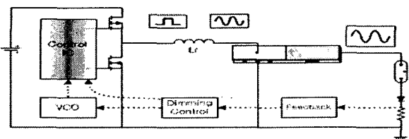
그림 5 하프-브리지 압전 인버터 Fig. 5 Half-Bridge Piezoelectric Inverter
