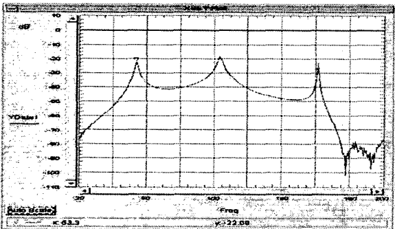
그림 1 압전 변압기의 전압전달특성 Fig. 1 Voltage Transfer Characteristics of the PT
