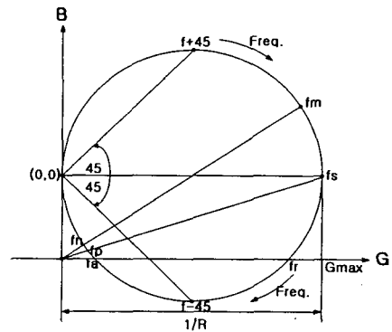
그림 2 어드미턴스 궤적법
