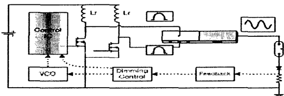
그림 4 푸시-풀 압전 인버터 Fig. 4 Push-pull Piezoelectric Inverter
