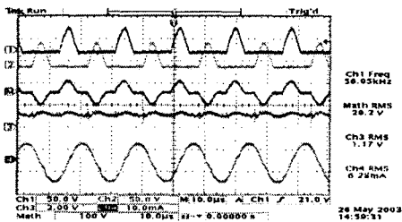
그림 10 최대휘도(푸시-풀) Fig. 10 Max. Brightness(Push-pull)
