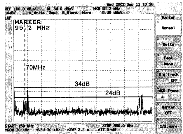
그림 2-13. Brushless DC 전동기의 노이즈 파형 Fig 2-13. Noise spectrum of BLDC motor
