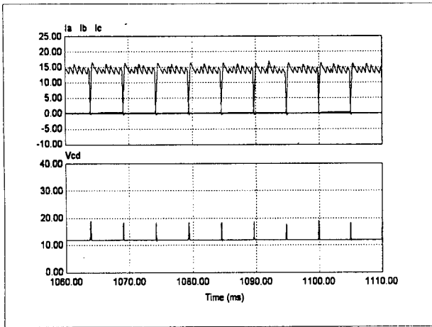
그림 2-7. Energy efficient C-dump 컨버터를 이용한 SRM의 3상전류 중첩파형 및 dump C 전압(1000rpm) Fig 2-7. 3phase-overlap waveforms and dump C voltage(1000rpm) by Energy efficient C-dump converter (Y축 : A, V, X축 : 시간(sec))
