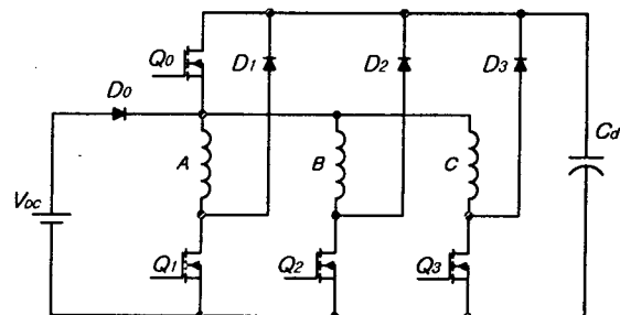
그림 2-1. Modified C-dump 컨버터 Fig 2-1. Modified C-dump converter
