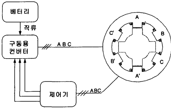
그림 2-4. 6/4극 스위치드 릴럭턴스 전동기의 단면도 Fig 2-4. A cross section of 6/4 pole Switched reluctance motor
