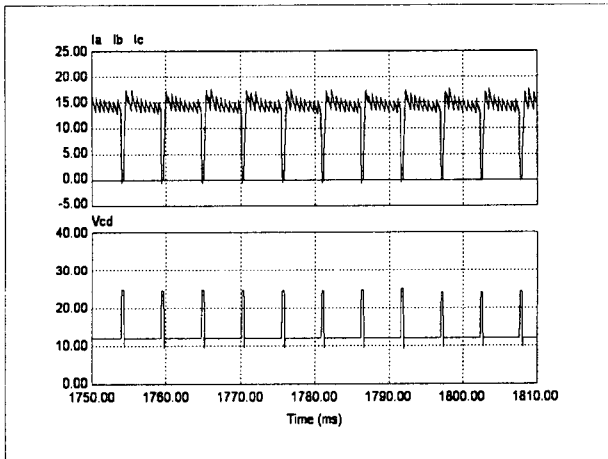
그림 2-8. Modified C-dump 컨버터를 이용한 SRM의 3상전류 중첩파형 및 dump C 전압(1000rpm) Fig 2-8. 3phase-overlap waveforms and dump C voltage(1000rpm) by Modified C-dump converter (Y축 : A, V, X축 : 시간(sec))
