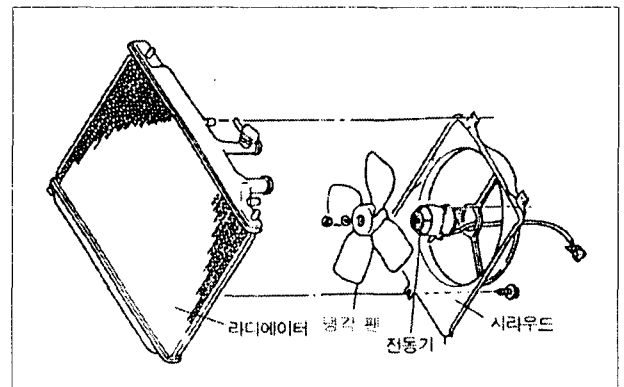
그림 2-3. 라디에이터 냉각 팬 Fig 2-3. Radiator cooling fan
