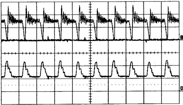
그림 2-11. Modified C-dump 컨버터를 이용한 SRM의 3상전류 중첩파형 및 dump C 전압(1000rpm)
