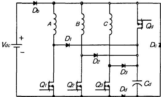
그림 2-2. Energy efficient C-dump 컨버터 Fig 2-2. Energy efficient C-dump converter
