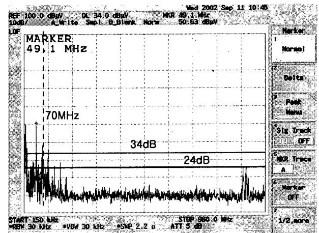
그림 2-14. DC 전동기의 노이즈 파형 Fig 2-14. Noise spectrum of DC motor
