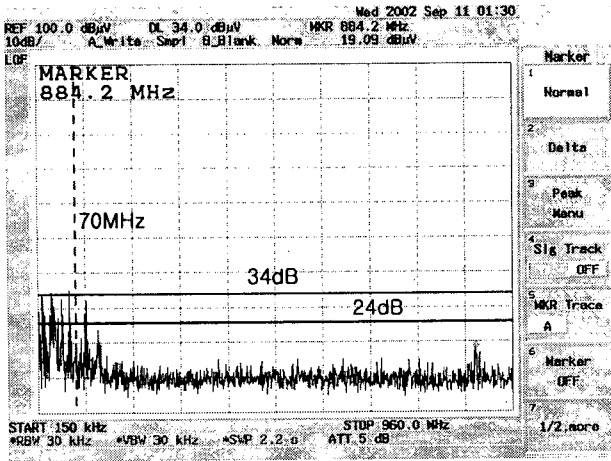
그림 2-15. 스위치드 릴럭턴스 전동기의 노이즈 파형 Fig 2-15. Noise spectrum of SRM
