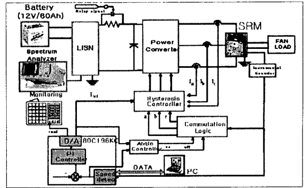
그림 2-9. 전체 시스템 구성도 Fig 2-9. The overall block diagram
