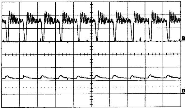
그림 2-10. Energy efficient C-dump 컨버터를 이용한 SRM의 3상전류 중첩파형 및 dump C 전압(1000rpm)
