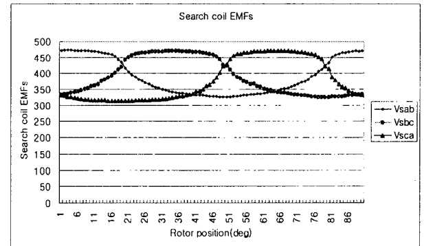
그림 5 회전자 위치에 따른 서치 코일 유기 기전력 분포 Fig. 5 Search coil EMFs according to the Rotor Position
