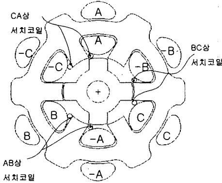
그림 1 Toroidal SRM과 서치 코일 Fig. 1 TSRM and Search coils
