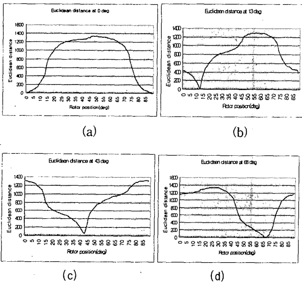
그림 6. 유클리디안 거리를 이용한 회전자의 위치 추정:
