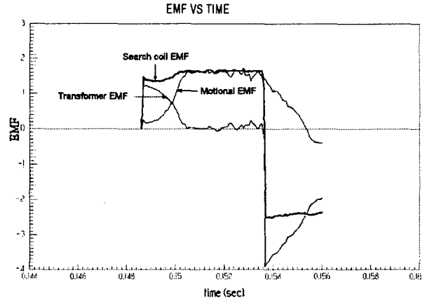
그림 3 서치 코일 파형의 성분 분석 Fig. 3 Analysis of waveform of a search coil
