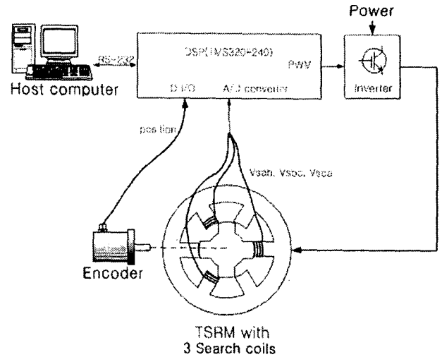
그림 7 전체 시스템 구성도
