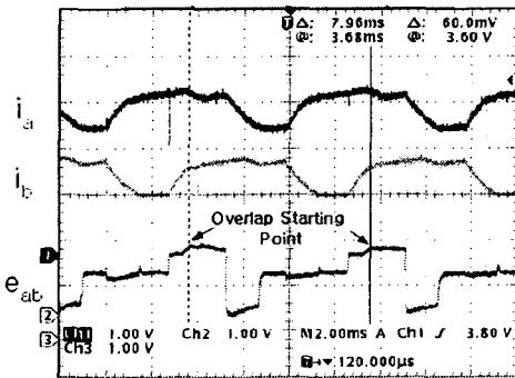
그림 2 A상, B상 전류와 AB 서치 코일 Fig. 2 Currents of A and B-phase and AB-search coil EMF
