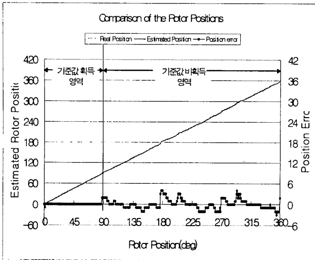
그림 8 추정된 회전자 위치와 실제 회전자 위치의 비교 Fig. 8 The comparison of the estimated rotor position and the real rotor position
