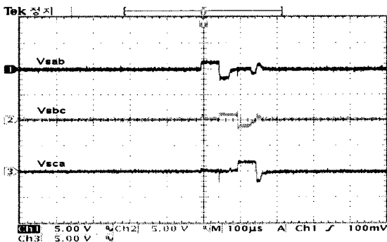
그림 4 단일펄스 입력에 대한 서치 코일 기전력 Fig. 4 Magnitude of the search coil EMFs
