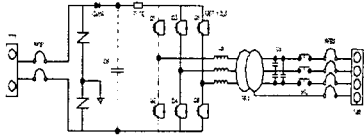
그림 3 인버터 전력회로도
