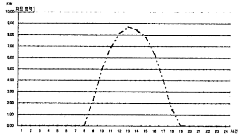
그림 7 태양전지 출력
