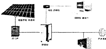
그림 1. 10kW급 태양광발전 시스템 구성도
