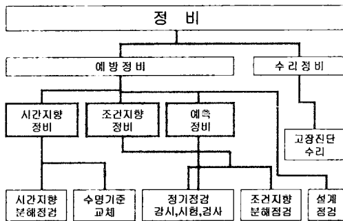
Fig 1 정비업무 형태
