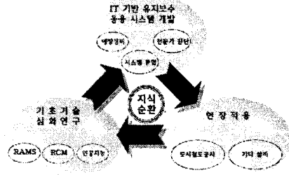
Fig 2 시스템개발 방향
