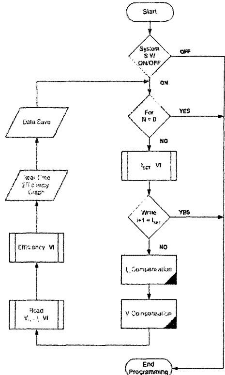
그림 3 효율 측정 시스템의 프로그램 흐름도
