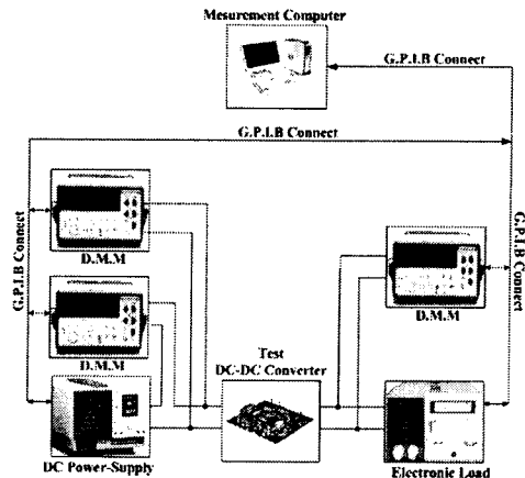
그림 1 효율 측정 시스템의 구성방법
