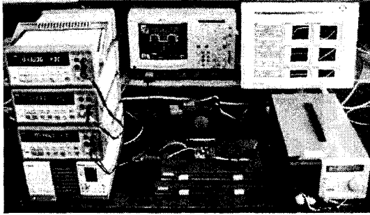
그림 2 효율 측정 시스템의 구성 사진
