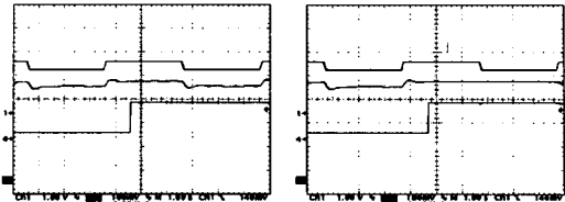
(a) 관성추정을 하는 경우 (b) 관성추정을 하지 않은 경우 그림 3. 속도 응답, 관성 추정 응답(실험 결과); 지령값, 추정값, 관성계수값 (관성계수 변화, 0.25*Jm)
