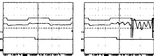
(a) 관성추정을 하는 경우 (b) 관성추정을 하지 않은 경우 그림 3. 속도 응답, 관성 추정 응답(실험 결과); 지령값, 추정값, 관성계수값 (관성계수 변화, 4*Jm)
