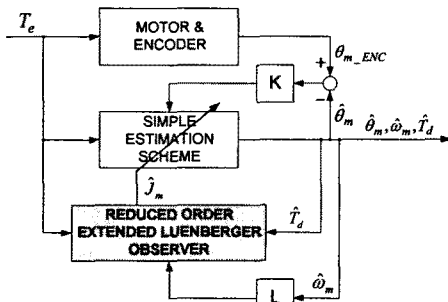
그림 1. 간략화한 추정기 블록도
