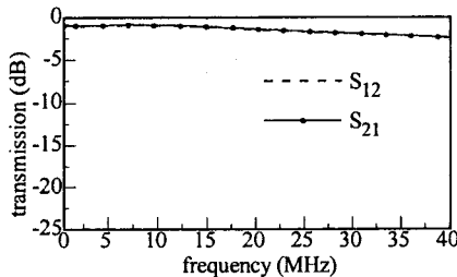
그림 4. 저압 전력선 결합기의 투과 특성.
