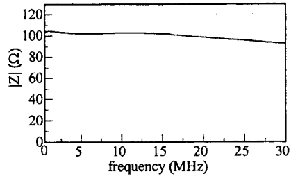
그림 5. 가변저항 측정결과.
