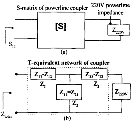
그림 2. 옥내 저압 회로망의 등가회로. (a) 저압 회로망. (b) 등가회로.
