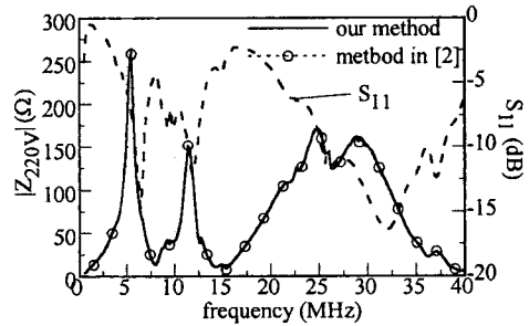
그림 6. 본 논문에서 제시한 방법과 참고문헌 [7]의 임피던스 측정 방법을 비교한 결과. S_{11} 은 그림 2(a)의 회로망 전체 반사계수.
