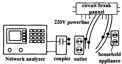
그림 1. 옥내 저압 전력선 배선망 및 임피던스 측정 Setup.
