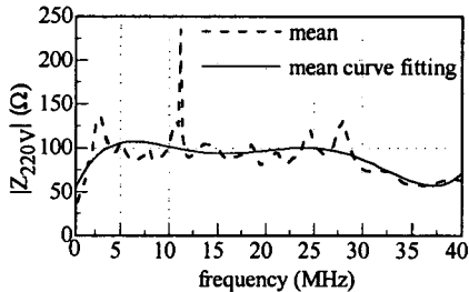
그림 7. 전체 아파트의 임피던스 산술 평균값과 산술 평균값의 다항식 curve fitting 결과.
