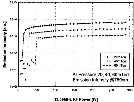
그림 3. Ar Gas 압력과 RF 전력 변화에 따른 Ar-I 라인인 750nm의 emission intensity Fig 3. Emission intensity (Ar-I 750) as a function of RF power variation for each gas pressure
