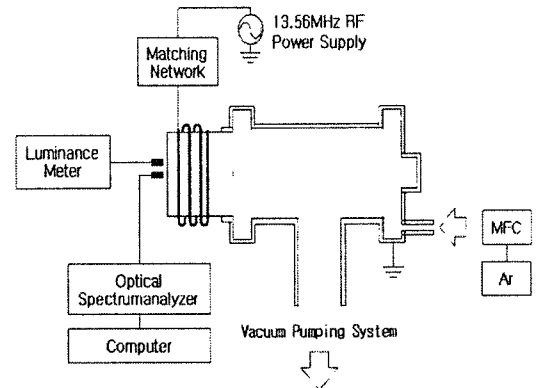
그림 1. 실험장치 개략도
