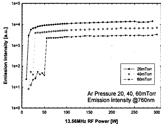
그림 4. Ar Gas 압력에서 RF 전력 변화에 따른 Ar-I 라인인 760nm의 emission intensity Fig 4. Emission intensity (Ar-I 760) as a function of RF power variation for each gas pressure
