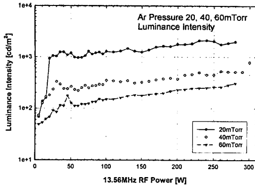
그림 5. Ar Gas 압력에서 RF 전력 변화에 따른 Ar-I 라인인 750nm의 휘도 측정 Fig 5. Luminance (Ar-I 750) as a function of power variation
