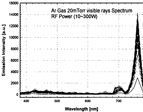
그림 2. Ar Gas의 Spectrum Fig 2. Spectrum Data of Ar Gas
