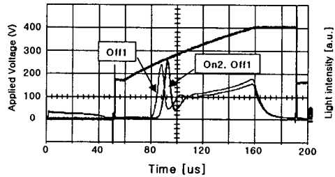
그림 5. sustain 650us인 파형, 15분간 방전후 on1, off1, off2의 광파형
