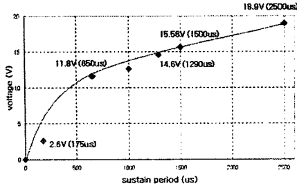
그림 7. sustain period 길이에 따른 on1과 off1의 광파형 peak치 전압차
