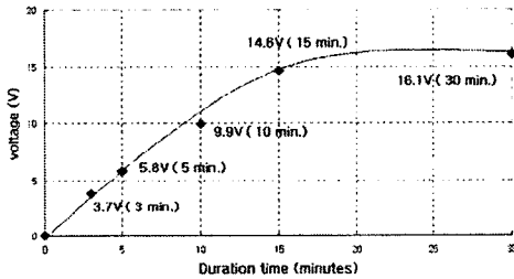
그림 8. 방전 지속 시간의 변화에 따른 on1과 off1의 광파형 peak치 전압차
