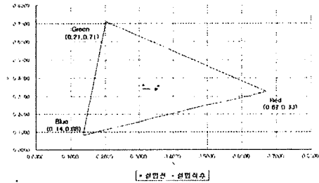
그림 11. Blue, Green cell만 방전 후 색좌표 이동
