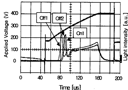
그림 6. sustain 2500us인 파형, 15분간 방전후 on1, off1, off2의 광파형
