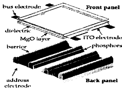
그림1. AC PDP의 개략도
