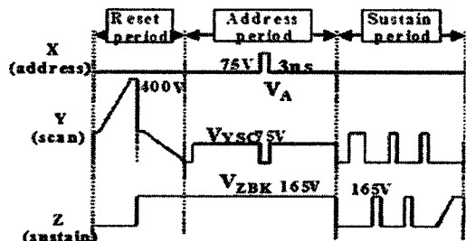
그림2. ADS 방식의 AC PDP 구동파형
