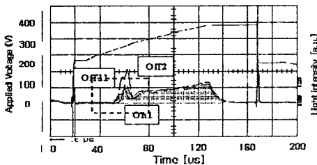
그림 9. Blue, Green 구동 후 전극 위치별 광파형
