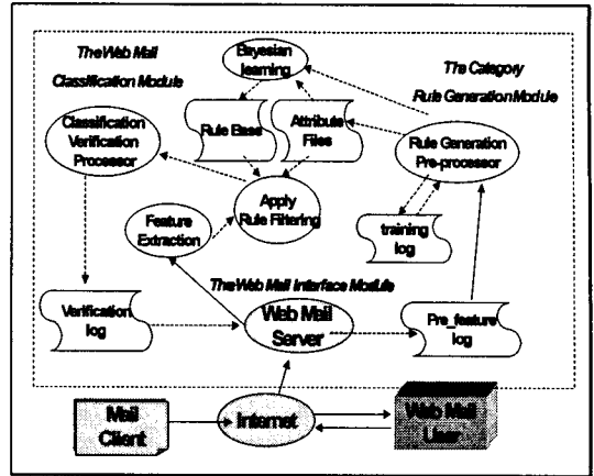
그림 2. WMP 에이전트 전체 구성도
