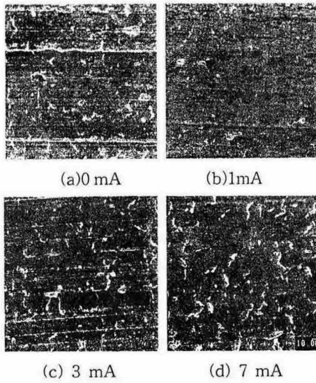
Fig. 7 Photo. of the rubbed surface for 3kg. (a) 0 mA, (b) 1 mA, (c) 3 mA, (d) 7 mA
