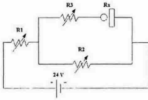
Fig. 2 전류인가 회로의 개요도
