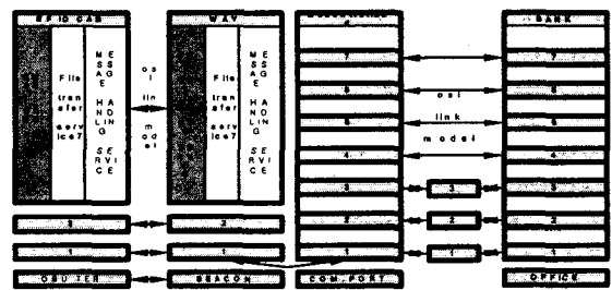
[그림 2] 도로측과의 통신 프로토콜 [Fig.2] Communication protocol side by road
