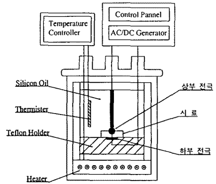
그림 1. 실험장치.
