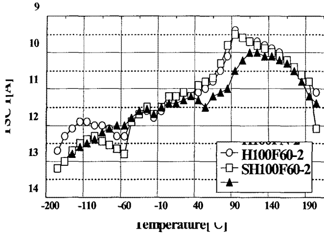
그림 4. 충전제 첨가 및 실란 처리에 따른 TSC 스펙트라.
