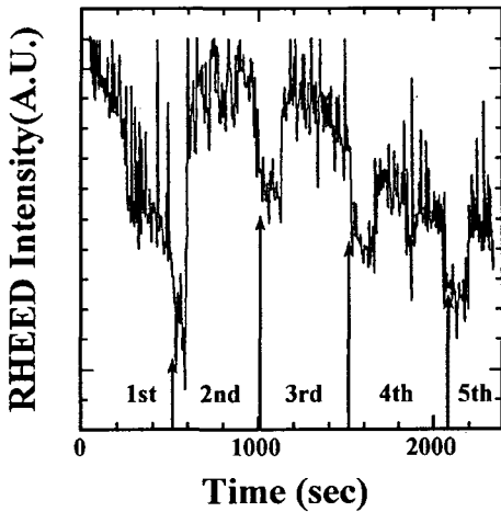
그림 3. RHEED 반사 스폿의 진동 Fig. 3. Variation of RHEED Intensity.
