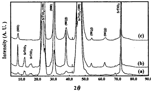
그림 1. 산화가스 압력에 따른 생성막의 결정 구조 변화
