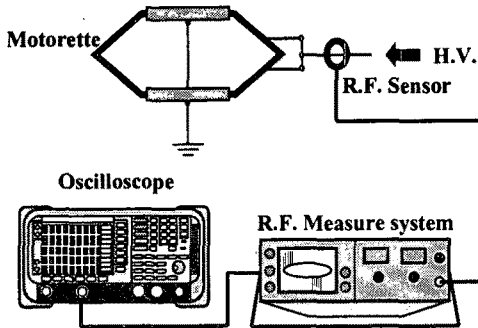
그림 1. HFPD 측정 시스템. Fig. 1. HFPD measurement system.
