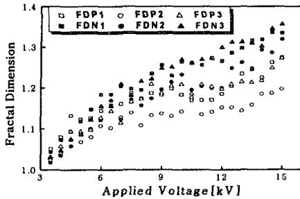
그림 5. 인가전압에 따른 프랙탈 차원 변화. Fig. 5. The change of fractal dimension according to applied voltages.
