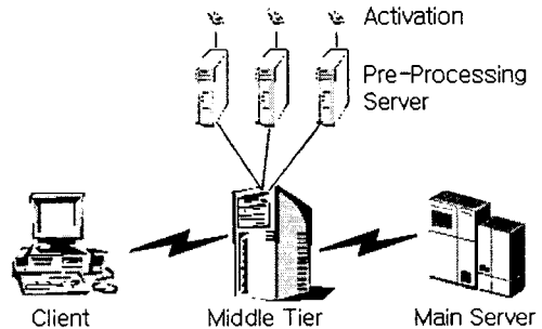
그림 5. Object Activation
