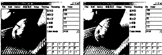
그림 7. Median
