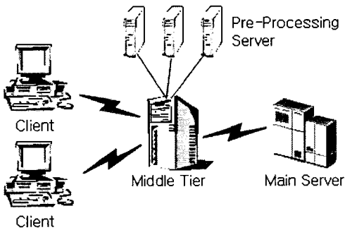
그림 4. Distributed Filtering
