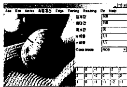
그림 8. Contrast
