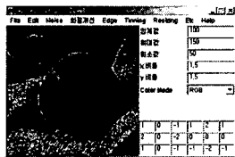
그림 10. Sovel
