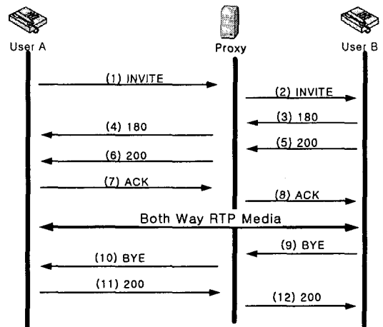
[그림2] SIP Call Flow
