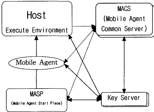
그림 2. MA 보안시스템의 구성도
