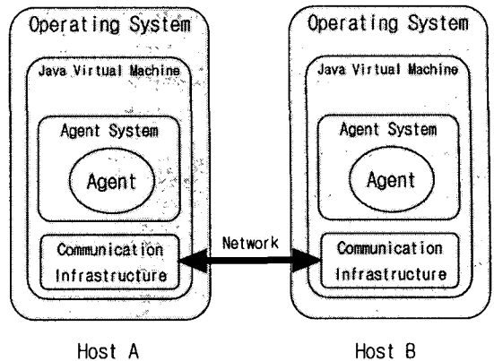
그림 1. Mobile Agent 모델
