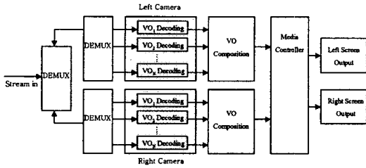
그림5. 입체 영상을 위한 Dual 스트림 디코더 개념도
