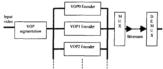
그림4. MPEG-4 인코더 기본 구조
