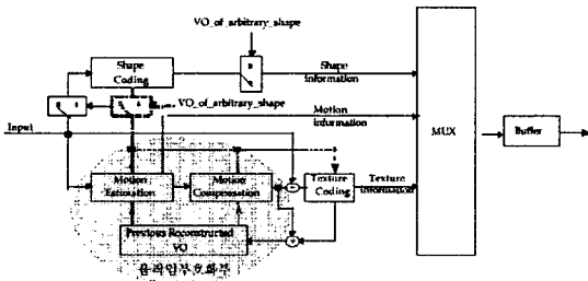
그림6. 입체 영상을 위한 Dual 스트림 MPEG-4 VOP 인코더 블록도
