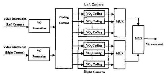
그림4. 입체 영상을 위한 Dual 스트림 인코더 개념도
