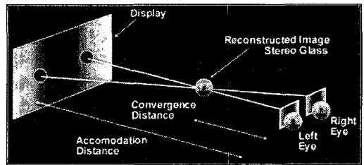
그림1. 스테레오스코픽(Stereoscopic)의 원리
