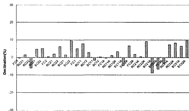
그림 18. 3차 장력계측값과 계산값의 차이
