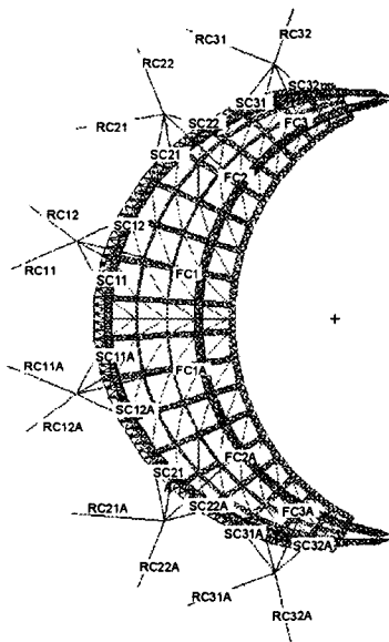
그림 2. 케이블 명칭
