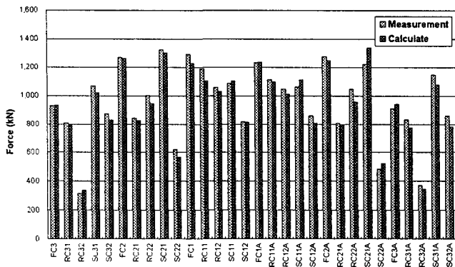
그림 17. 3차 장력계측 결과
