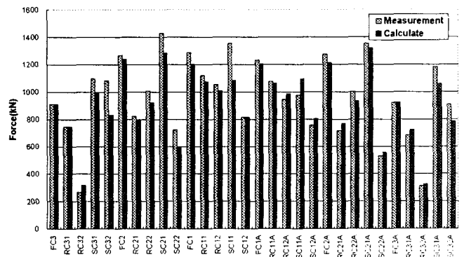
그림 15. 2차 장력계측 결과
