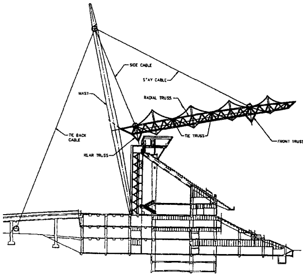
그림 1. 제주월드컵경기장 단면도
