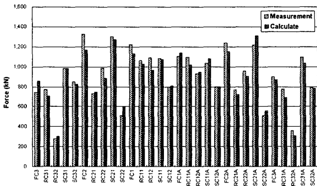
그림 13. 1차 장력계측 결과
