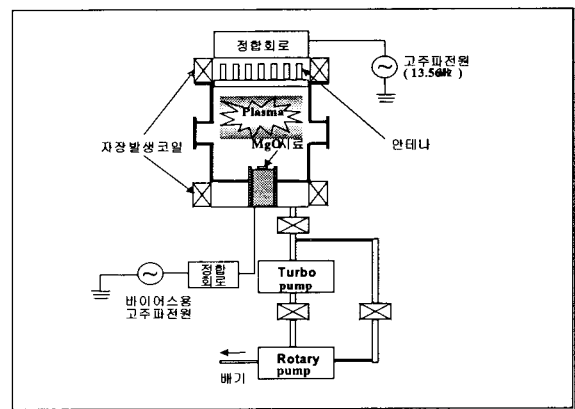
그림 1. 유도 결합형 플라즈마 식각 장치 Fig.1. Schematic diagram of Inductivity Coupled Plasma Etching System
