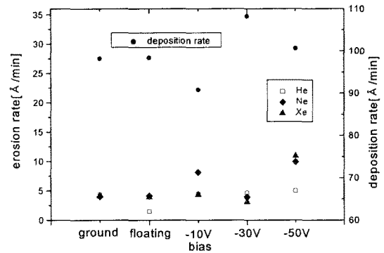
그림 3. bias전위에 따라 증착된 MgO의 deposition rate과 erosion rate Fig. 3. Deposition rate and erosion rate of MgO vs. bias voltage
