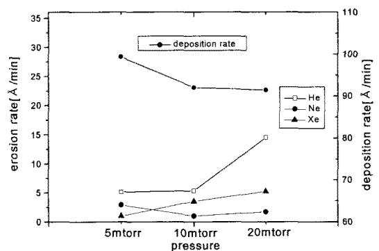
그림 4. 압력변화에 따라 증착된 MgO의 deposition rate과 erosion rate Fig. 4. Deposition rate and erosion rate of MgO vs. pressures
