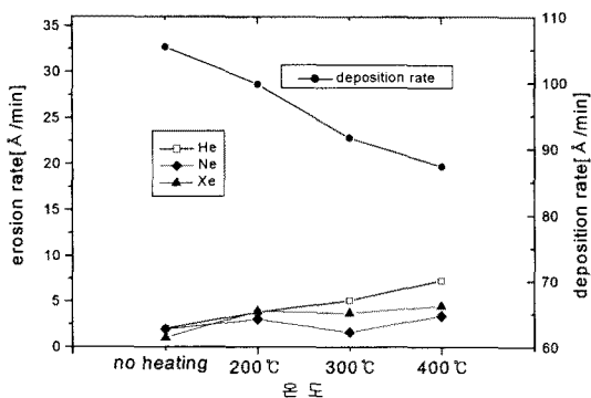
그림 2. 온도에 따라 증착된 MgO의 deposition rate과 erosion rate Fig. 2. Deposition rate and erosion rate of MgO vs. temperatures
