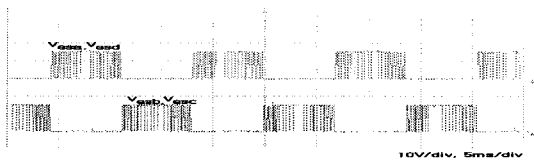
그림 11. 인버터 스위치 Sa, Sd와 Sb, Sc의 제어신호 Fig. 11. Control signal of inverter switch Sa, Sd and Sb, Sc
