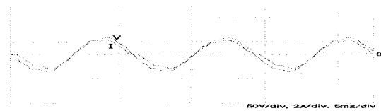
그림 7. 입력전압과 입력전류의 파형 Fig. 7. Waveform of input voltage and current
