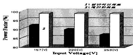
그림 12. 입력전압과 역률의 특성 Fig. 12. Characteristics of input voltage a power factor
