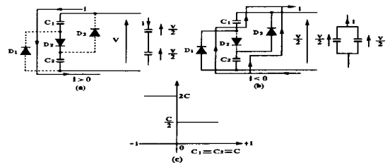
그림 2. 비선형 캐패시터의 회로 Fig. 2. Circuit of nonlinear capacitance
