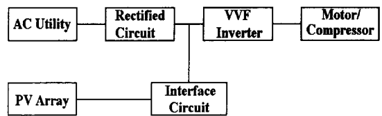
그림 1. 직류측 병렬 연계시스템 Fig. 1. Grid connected system with a rectifier
