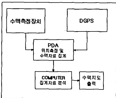
그림 1. 수맥탐사 시스템 구성도
