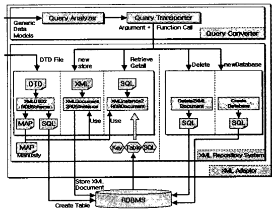
그림 2. XML 어댑터의 세부 구조
