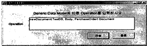
그림 6. 문서 생성을 위한 질의
