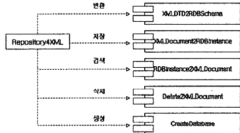
그림 5. XML 저장관리 시스템의 컴포넌트 다이어그램
