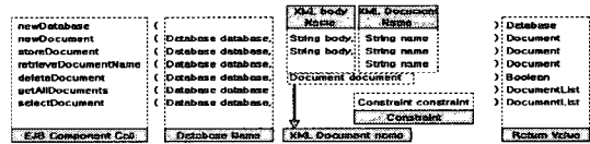
그림 5. Generic Data Model을 SQL로 변환 방법
