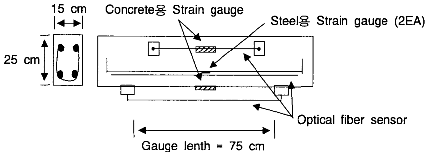
<그림 5> 철근매립부 변형률 측정을 위한 시험체(CTL I, II)
