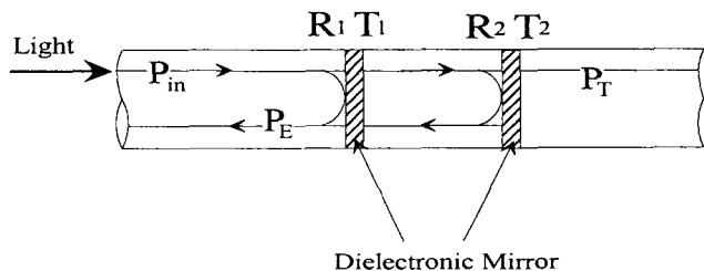
<그림 3> Fabry-Perot 광섬유 센서의 구조
