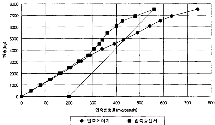
<그림 6> 전기저항식 게이지와 FBG 광섬유 센서의 압축변형률측정결과(CTL II)
