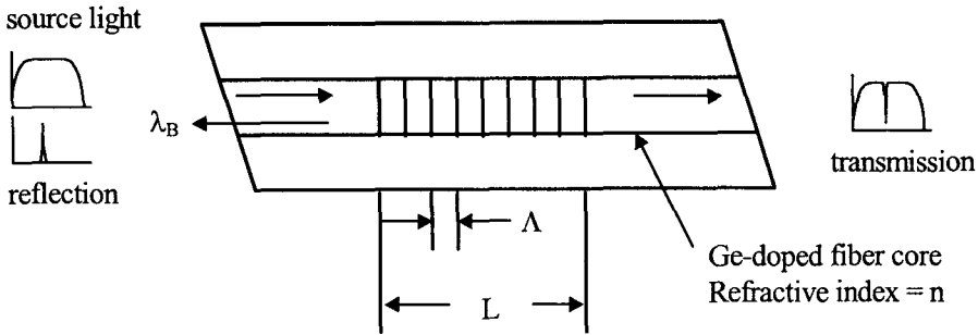
<그림 2> Fiber Bragg Grating 구조
