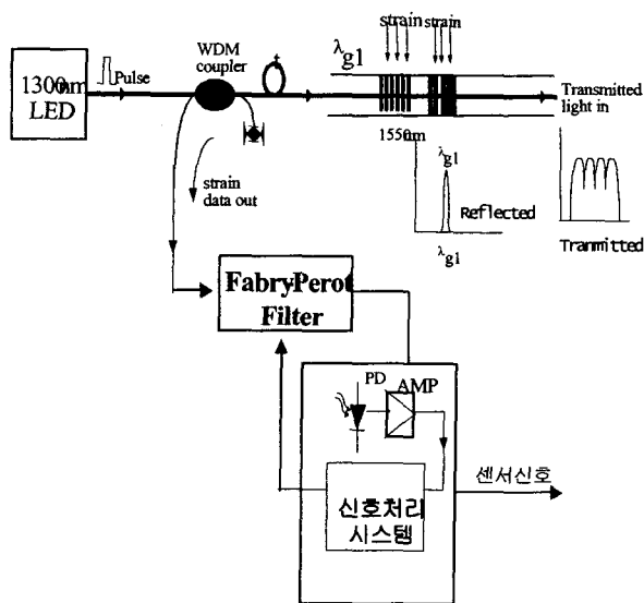
<그림 4> Fiber Bragg Grating Sensor System 전체 블럭도
