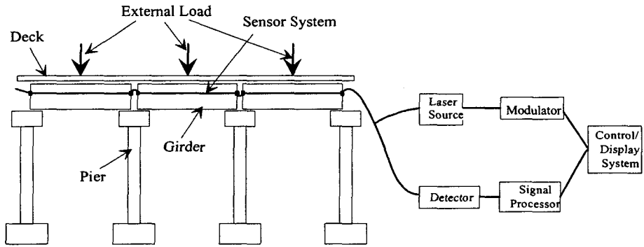
<그림 1> 광섬유를 이용한 교량 유지관리 시스템
